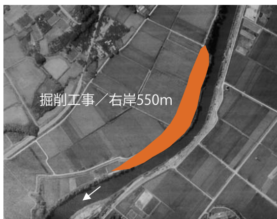
剣吉橋と穂並橋の間付近の右岸を掘削
