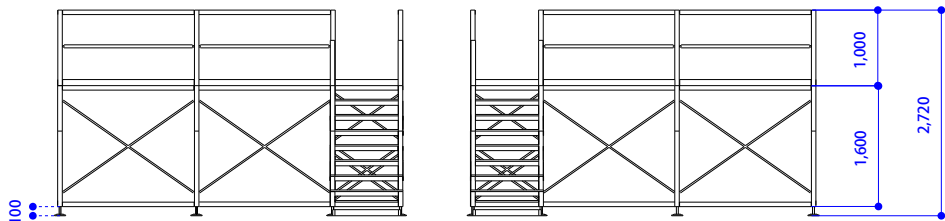
◇側面図
