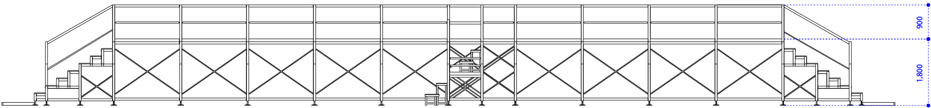
◇立面図
