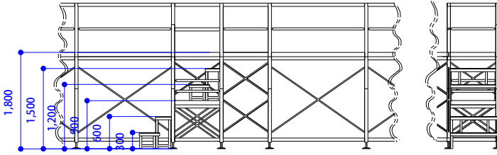
◇中央階段図
